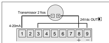
Figura 8 - Conexão de transmissor 2 fios com a fonte 24Vcc do controlador
