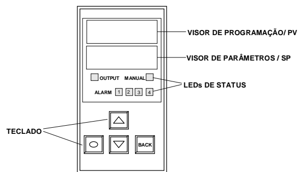
Figura 1 - Identificação das partes do painel frontal
