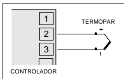
Figura 4 - conexão de termopar
