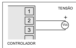
Figura 5 - conexão de tensão
