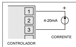
Figura 7 - conexão de corrente
