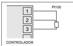
Figura 6 - conexão de Pt100 a 3 fios
