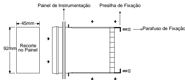
Figura 02 – Sistema de fixação
