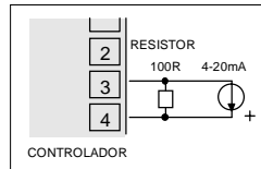
Figura 9 - Conexão para SP remoto
