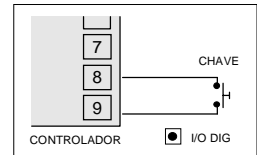
Figura 10 - Conexão de entrada digital
