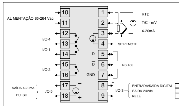
Figura 03 – Conexões do painel traseiro
